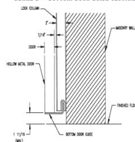
DETAIL D - BOTTOM DOOR GUIDE SECTION
